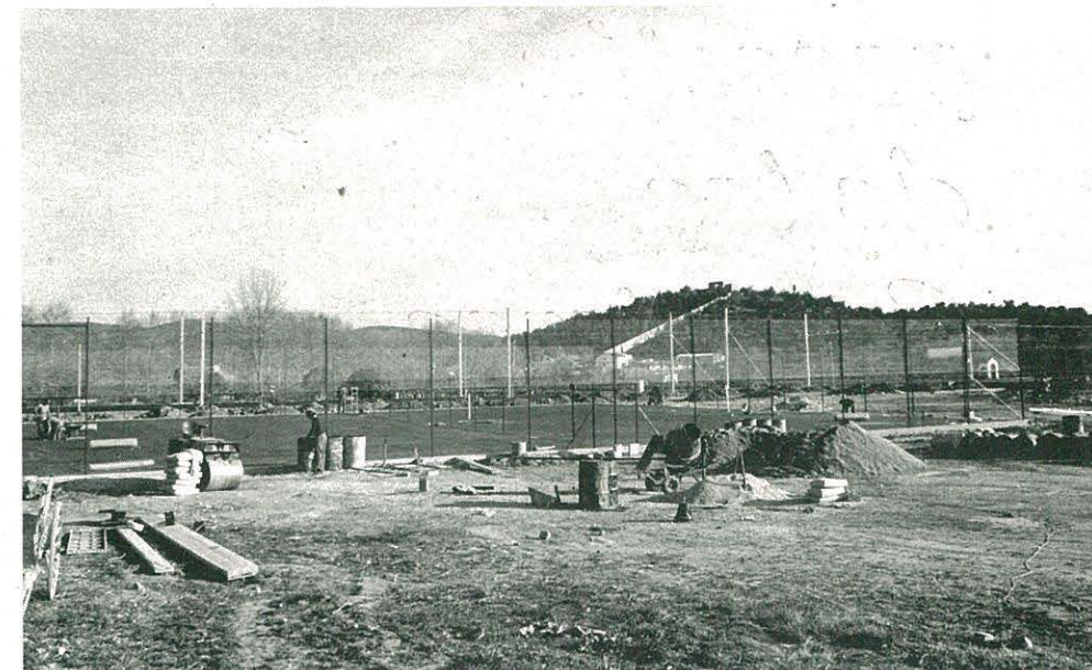
Montaje de la valla metálica y colocación de pavimentos en el terreno de juego.
