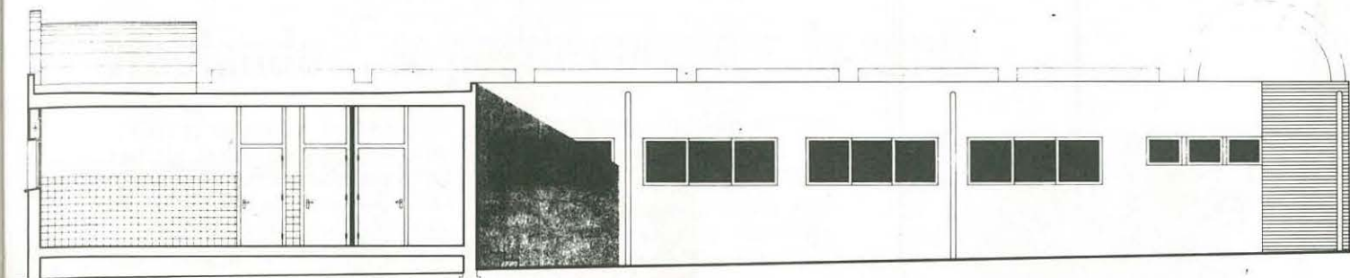
FAÇANA D-D
